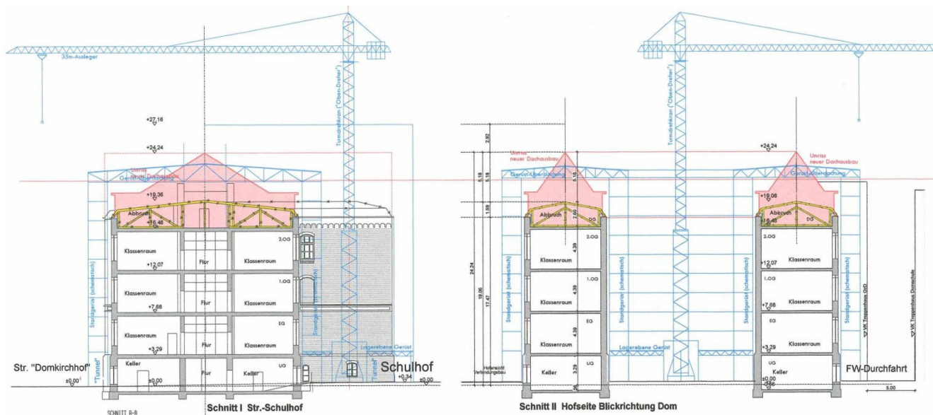
Schnitt + Baustelleneinrichtung
