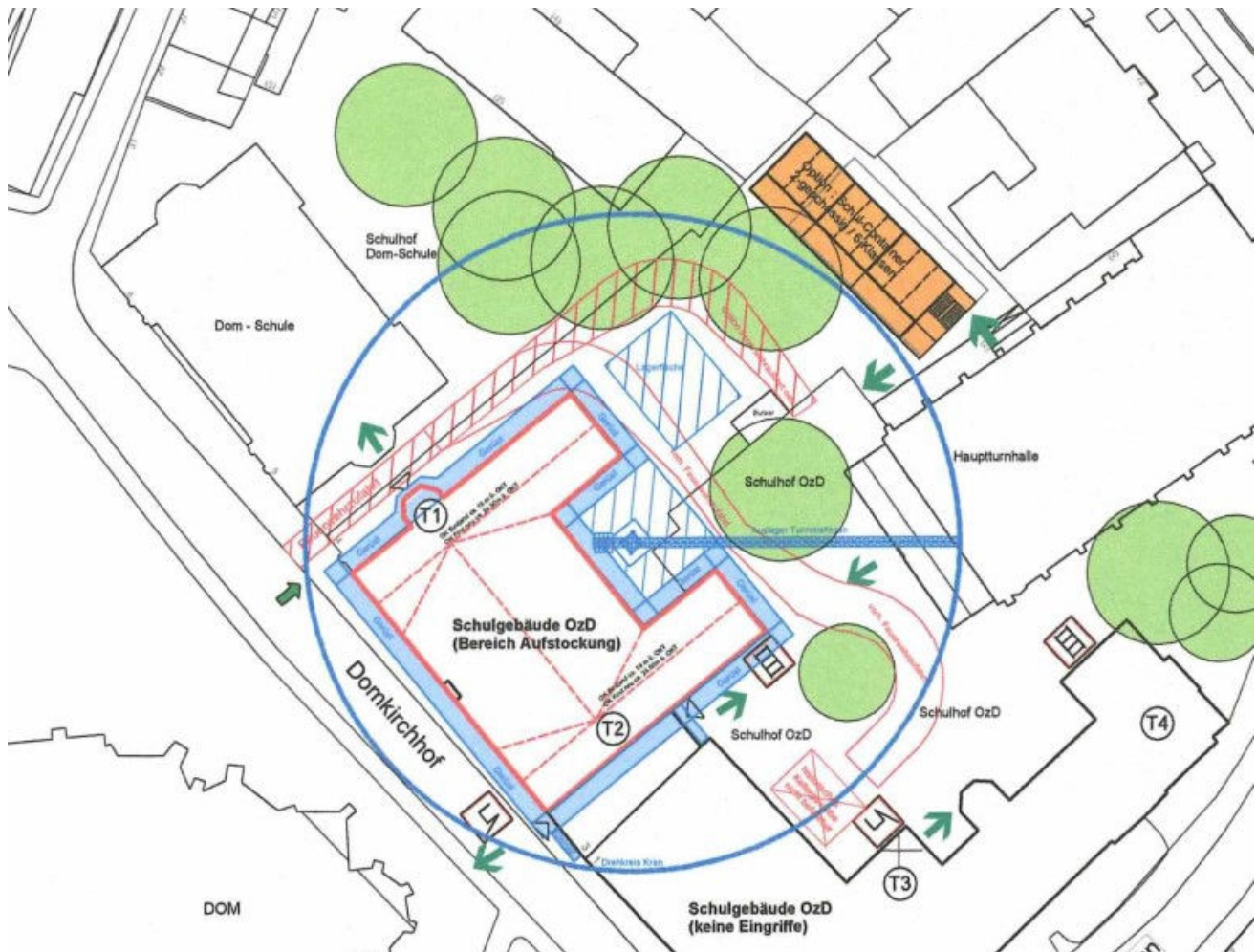
Lageplan + Baustelleneinrichtung
